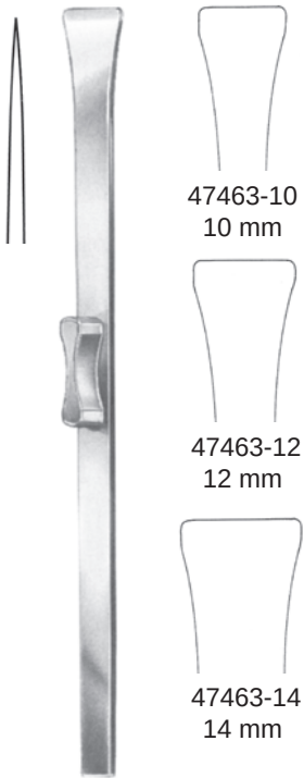
RUBIN 18,5 cm, 7 ¼"
