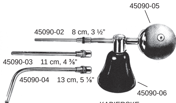
KABERSKE 45090-00 30 ccm komplett mit 3 Kanülen und Gummiball complete with 3 cannulas and rubber bulb completo con 3 cánulas y pera de goma
